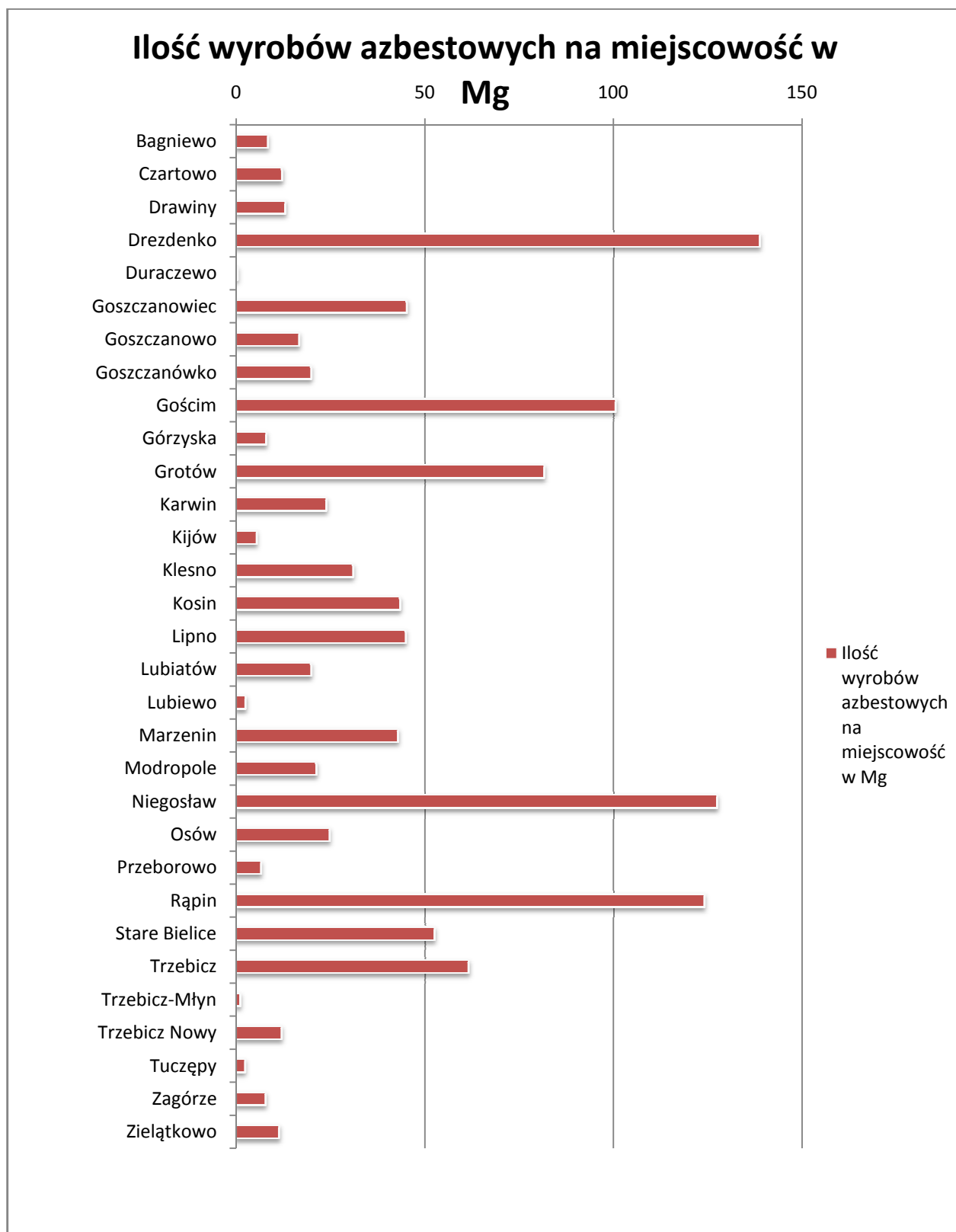
Wykres nr 2. Ilość wyrobów azbestowych w Mg w miejscowościach
