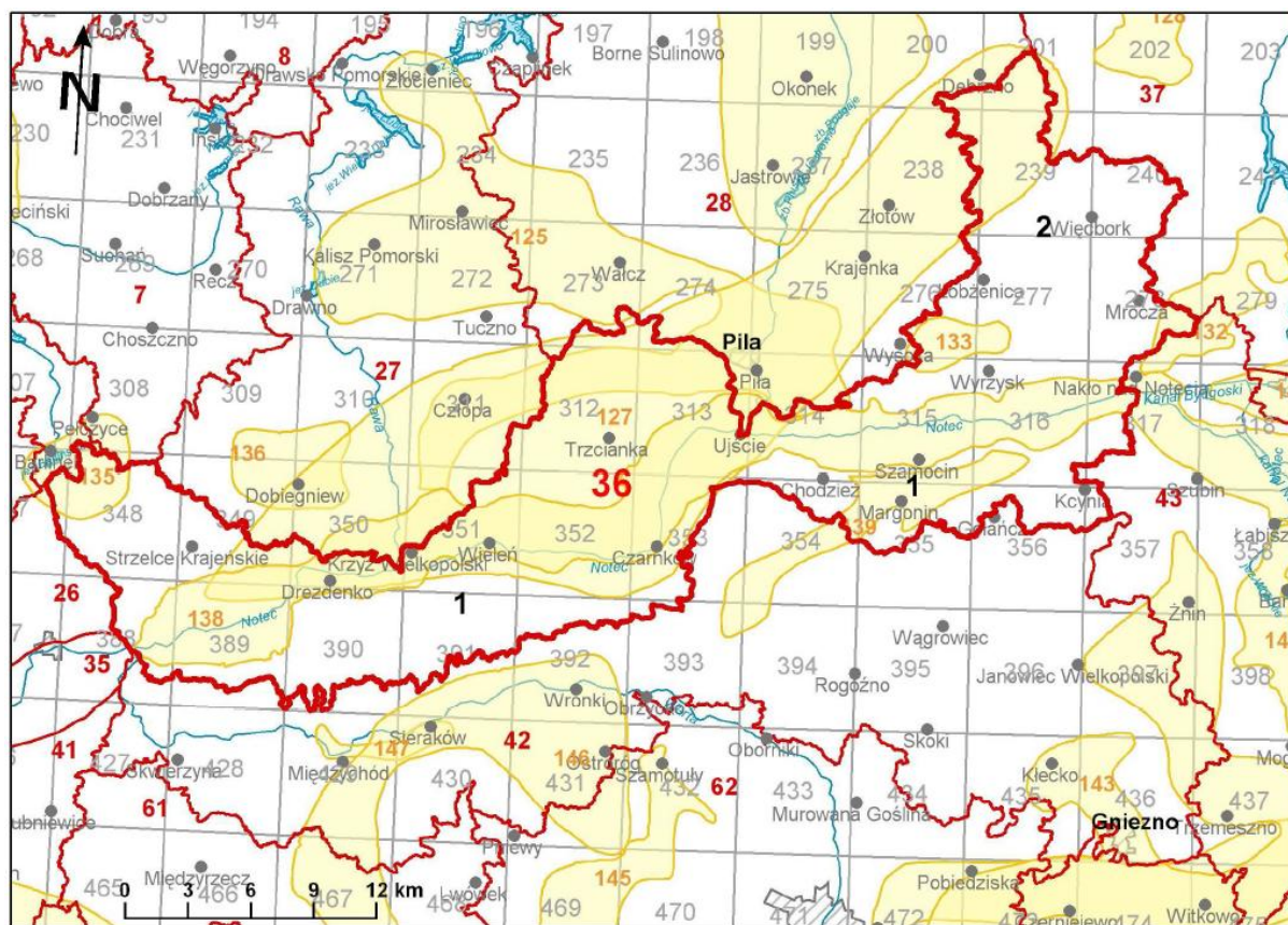
Lokalizacja GZWPd
